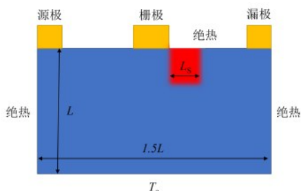
图5 二维晶体管模型
