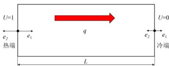
图3 一维热传导问题
