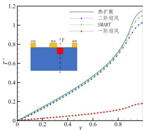
(b) X=0.755 上温度的分布
