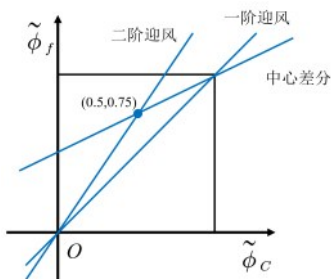
图11 规正变量图
