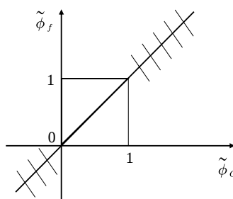
图12 对流有界性准则
