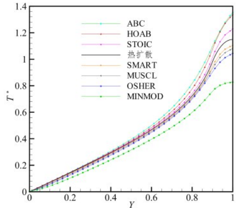
图 16 高阶有界格式的结果
