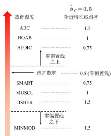
图 17 不同格式计算的热源温度排序
