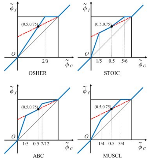
图 15 OSHER、STOIC、ABC 与 MUSCL 格式的特征线
