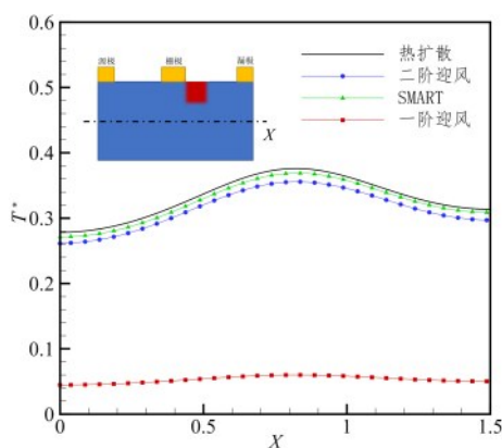
(a) Y=0.5 上温度的分布
