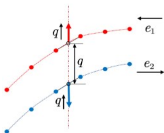
图13 界面值偏差对热流计算的影响
