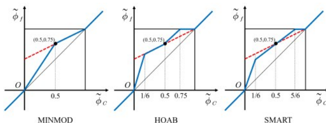
图14 MINMOD、HOAB与SMART格式的特征线
