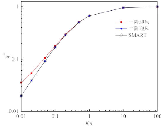
(b) 不同 Kn 下的无量纲热流
