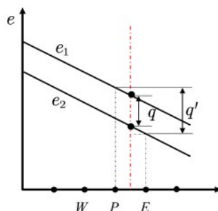
图7 偏置误差
