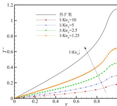
图8 网格疏密程度对偏置误差的影响
