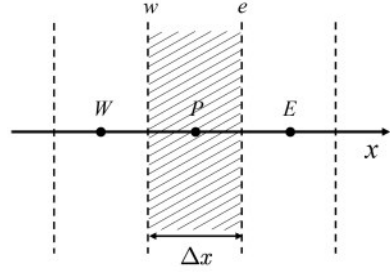
图2 一维控制体示意图
