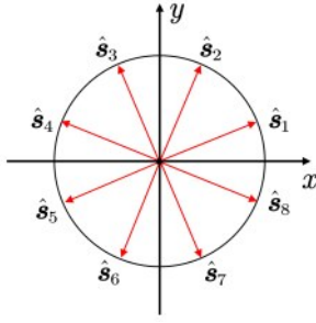
图1 一种速度方向离散格式
