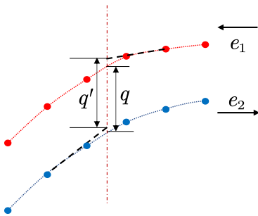
图9 非线性分布的偏置误差 Fig. 9 Offset error of nonlinear distribution
